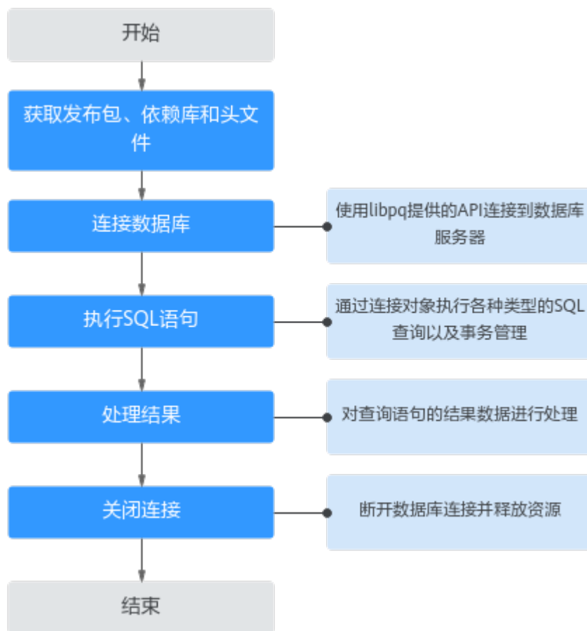
图 5-3 libpq 开发流程图
