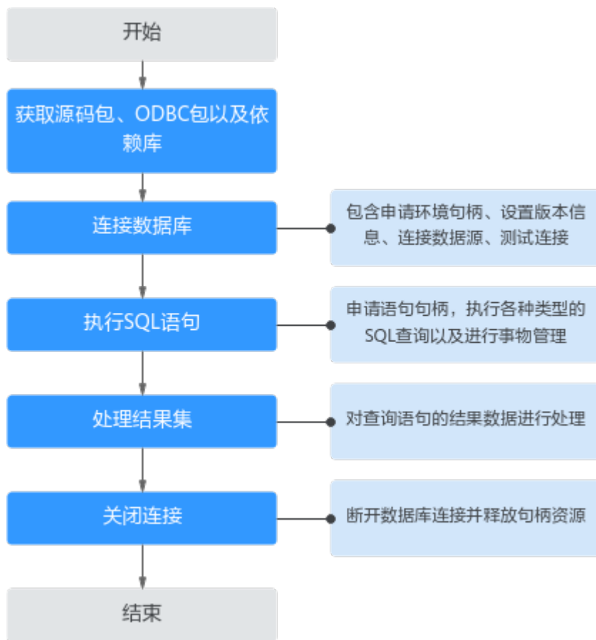
图 5-2 ODBC 开发流程图
