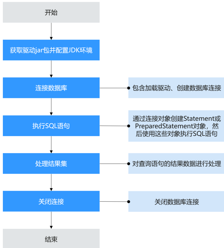
图 5-1 采用 JDBC 开发应用程序的流程
