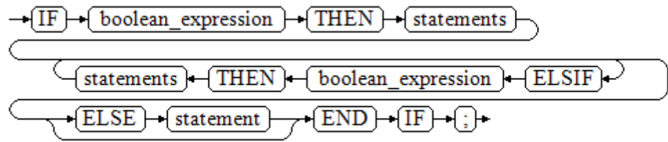
图 10-17 IF_THEN_ELSIF_ELSE::=
