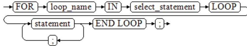
图 10-33 FOR_AS_loop::=
