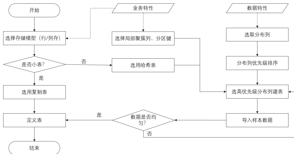
图 6-2 表定义流程
