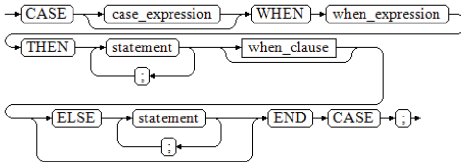
图 10-23 case_when::=
