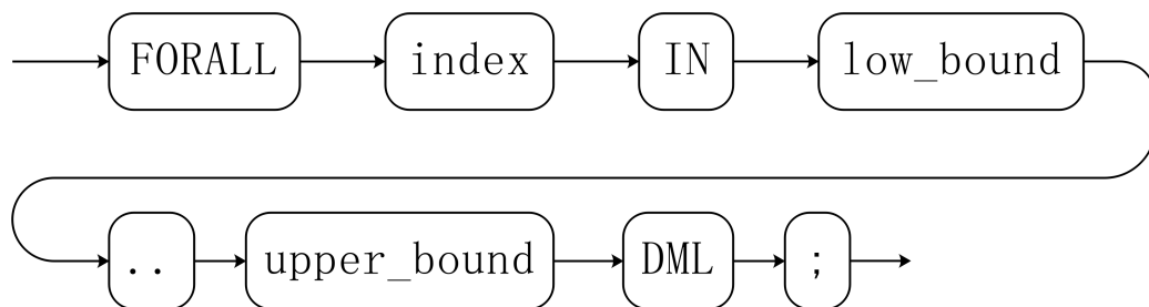
图 10-22 forall::=
