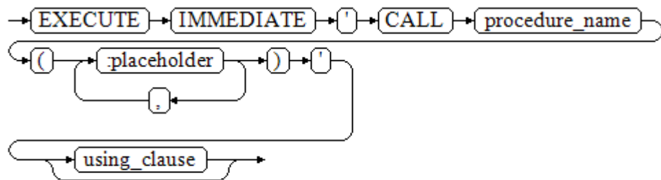
图 10-10 call_procedure::=
